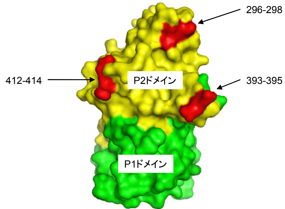
図5 P2ドメインにおけるVariant Specific Epitope 本図の下部にSドメインの構造を加えたタンパク質モノマー2つで組織されたダイマーカプソメア（2量体）が、90個組み合わせあって正20面体のウイルス粒子を構成する。
